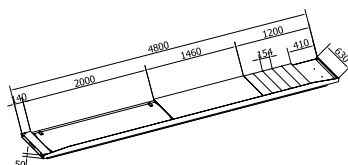
Pasarela de alineación Alignment platform Passerelle géométrie
