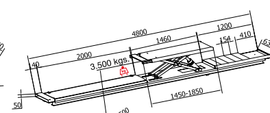
Pasarela de alineación con elevador auxiliar hidráulico Alignment platform with hydraulic wheel free (aux. lift table) Passerelle géométrie avec relevage auxiliaire hydraulique (lift table)
