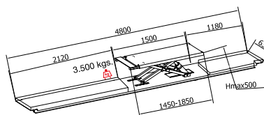
Pasarela lisa con elevador aux. hidráulico integrado Flat platform with hydraulic wheel free (aux. lift table integrated) Passerelle lisse avec relevage auxiliaire hydraulique (lift table intégré)
