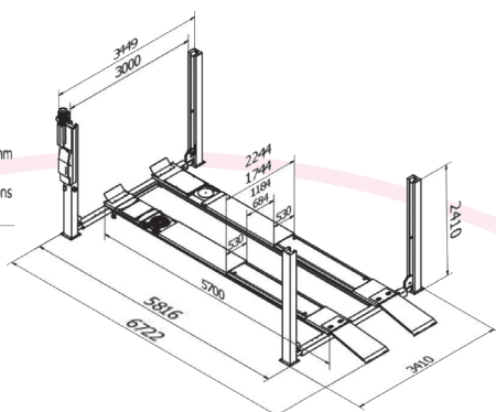
Rampes SPORT disponibles Réf. 33750
