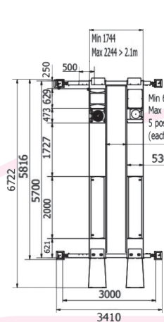
Rampes SPORT disponibles Réf. 33750
